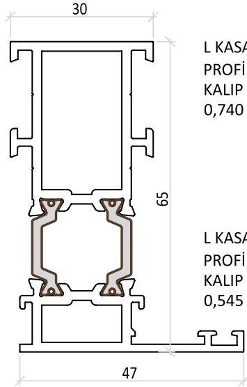
L KASA PROFİLİ KALIP NO 65002 1,285kg/mt Jx: 25,5 cm 4 Jy: 5,46 cm 4
