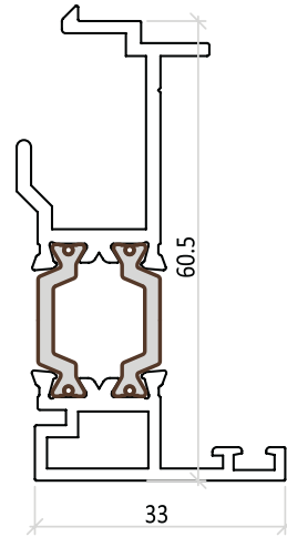
İÇE-ÇİFT KANAT ADAPTÖR PR. (İÇ) KALIP NO: 5726 0,438 kg/mt
