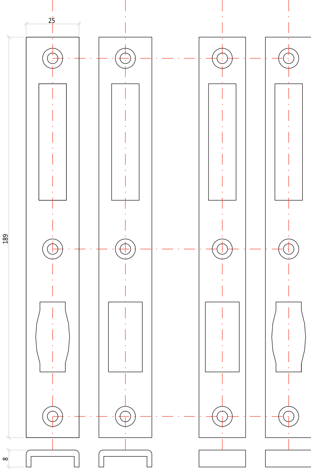
U KİLİT KARŞILIĞI
