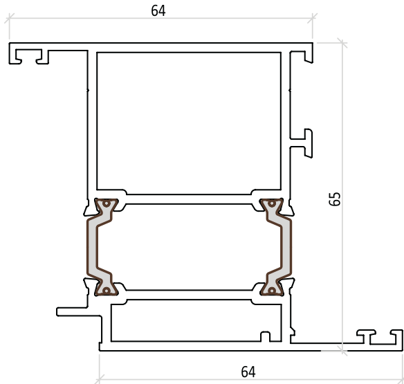
İÇE-DIŞA KANAT PROFİLİ (İÇ) KALIP NO: 5723 1,005 kg/mt
