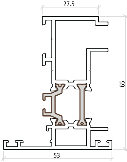
ÇİFT KANAT ADAPTÖR PROFİLİ KALIP NO 65010 1,227 kg/mt Jx: 24,24 cm 4 Jy: 5,89 cm 4
