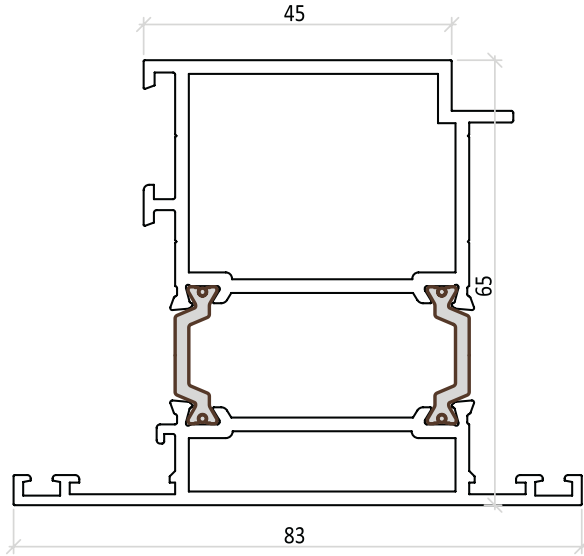
İÇE-DIŞA KANAT PROFİLİ (İÇ) KALIP NO: 5721 0,939 kg/mt
