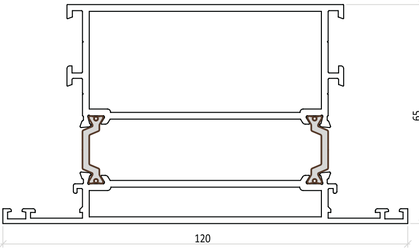
ALT ETEK PROFİLİ KALIP NO 65017 2,534 kg/mt Jx: 83,02 cm 4 Jy: 52,28 cm 4
