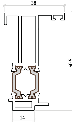
DIŞA-ÇİFT KANAT ADAPTÖR PROFİLİ (İÇ) KALIP NO: 5730 0,674 kg/mt
