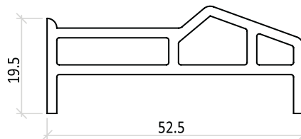
EŞİK PROFİLİ KALIP NO 5734 0,8 kg/mt
