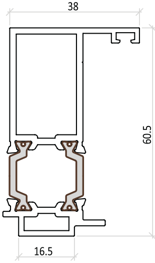
DIŞA AÇILIM ADAPTÖR PROFİLİ (İÇ) KALIP NO: 5728 0,674 kg/mt
