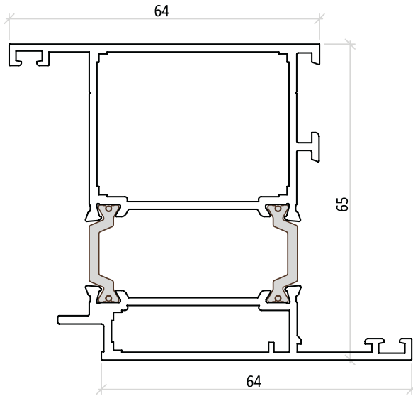
İÇE-DIŞA KANAT PROFİLİ (İÇ) KALIP NO: 5814 0,871 kg/mt
