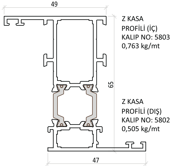
Z KASA PROFİLİ KALIP NO 65106 1,269 kg/mt Jx: 29,07 cm 4 Jy: 6,63 cm 4
