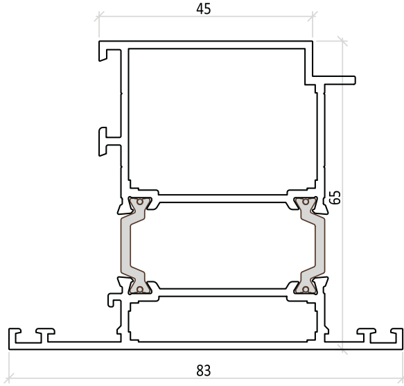
İÇE-DIŞA KANAT PROFİLİ (İÇ) KALIP NO: 5812 0,802 kg/mt
