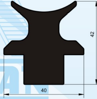
Profil No : 6029 Gramaj : 1.723 kg/m Çevre : 389 mm
