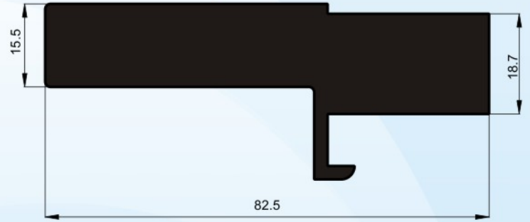
Profil No : 6019 Gramaj : 3.723 kg/m Çevre : 238 mm
