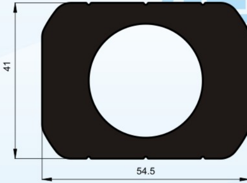
Profil No : 6018 Gramaj : 3.921 kg/m Çevre : 177 mm
