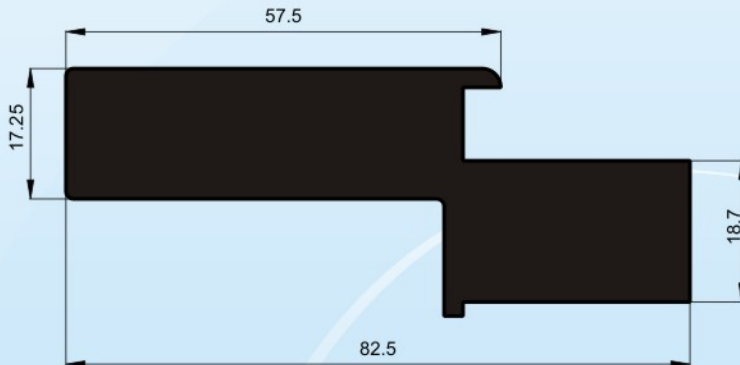
Profil No : 6020 Gramaj : 4.108 kg/m Çevre : 238 mm
