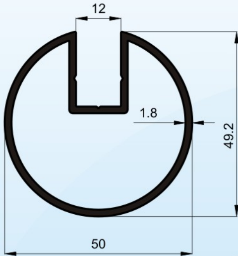
Profil No : 6119 Gramaj : 0.927 kg/m Çevre : 197 mm
