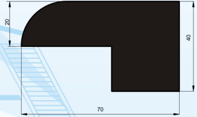
Profil No : 6017 Gramaj : 5.187 kg/m Çevre : 211 mm
