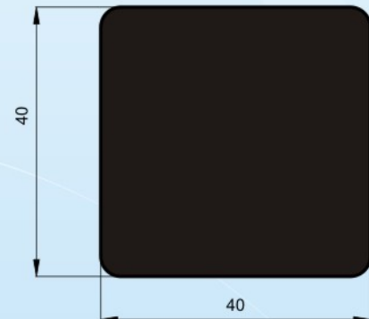
Profil No : 6031 Gramaj : 4.314 kg/m Çevre : 155 mm
