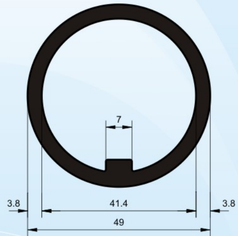
Profil No : 6149 Gramaj : 0.564 kg/m Çevre : 154 mm
