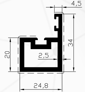
Profil No : 1903 Gramaj : 0.713 kg/m Çevre : 145 mm
