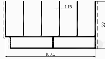
Profil No : 7150 Gramaj : 1.463 kg/m Çevre : 691 mm
