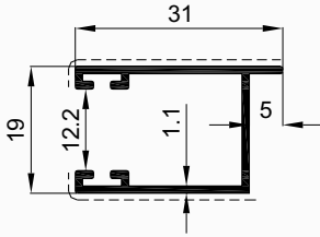
Profil No : 2648 Gramaj : 0.268 kg/m Çevre : 179 mm
