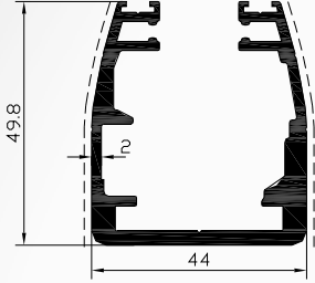
Profil No : 6162 Gramaj : 1.409 kg/m Çevre : 387 mm
