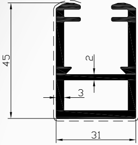
Profil No : 1901 Gramaj : 1.212 kg/m Çevre : 257 mm
