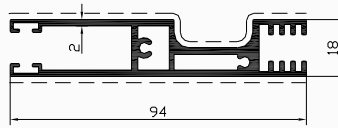
Profil No : 7153 Gramaj : 1.401 kg/m Çevre : 430 mm
