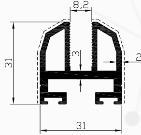
Profil No : 1902 Gramaj : 0.904 kg/m Çevre : 231 mm
