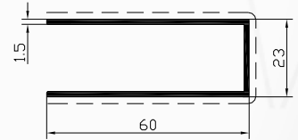
Profil No : 7154 Gramaj : 0.569 kg/m Çevre : 282 mm
