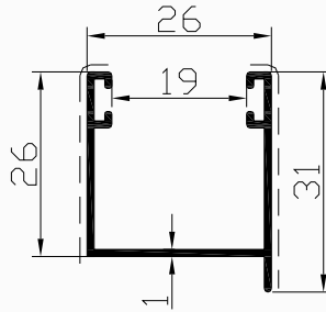
Profil No : 2244 Gramaj : 0.259 kg/m Çevre : 191 mm
