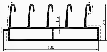
Profil No : 7152 Gramaj : 1.667 kg/m Çevre : 550 mm
