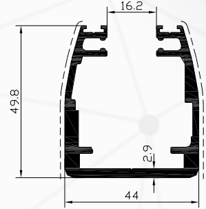
Profil No : 6164 Gramaj : 1.371 kg/m Çevre : 380 mm
