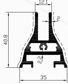
Profil No : 6163 Gramaj : 0.910 kg/m Çevre : 229 mm
