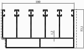
Profil No : 8741 Gramaj : 1.760 kg/m Çevre : 840 mm
