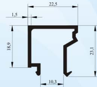
Profil No : 2594 Gramaj : 0.305 kg/m Çevre : 152 mm
