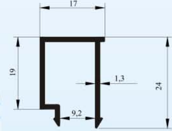
Profil No : 2583 Gramaj : 0.231 kg/m Çevre : 134 mm
