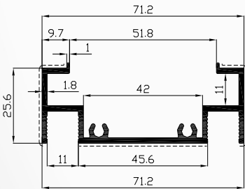
Profil No : 3590 Gramaj : 0.848 kg/m Çevre : 368 mm
