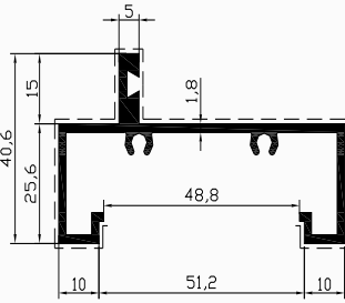
Profil No : 3587 Gramaj : 0.974 kg/m Çevre : 372 mm
