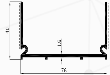
Profil No : 3589 Gramaj : 0.816 kg/m Çevre : 332 mm
