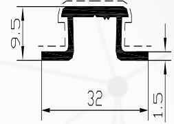
Profil No : 3586 Gramaj : 0.223 kg/m Çevre : 105 mm
