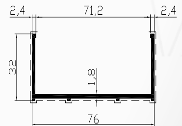
Profil No : 3592 Gramaj : 0.684 kg/m Çevre : 284 mm
