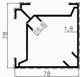
Profil No : 3591 Gramaj : 1.906 kg/m Çevre : 442 mm
