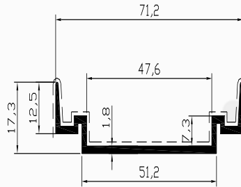
Profil No : 3588 Gramaj : 0.518 kg/m Çevre : 226 mm
