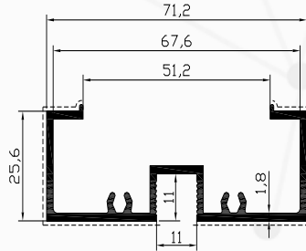
Profil No : 3585 Gramaj : 0.855 kg/m Çevre : 364 mm
