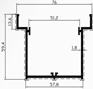
Profil No : 3584 Gramaj : 1.037 kg/m Çevre : 439 mm
