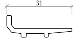
CAM TAKOZU PROFİLİ 5055 0,240 kg/m (Cam Kalınlığı 24mm'e Kadar)
