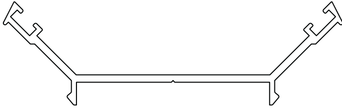
DIŞ KÖŞE ALT KAPAK 5101 0,825 kg/m
