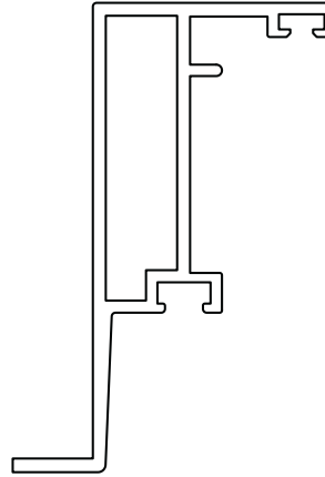
CEPHE İÇİ KANAT KASA PROFİLİ 5118 0,797 kg/m Jx: 12,57 cm 4 Jy: 1,38 cm 4
