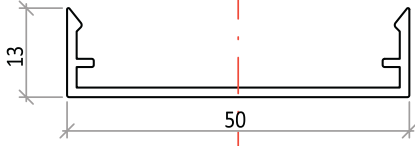
KAPAK PROFİLİ 5053 0,294 kg/m
