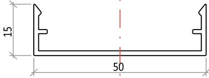
KAPAK PROFİLİ 5052 0,309 kg/m
