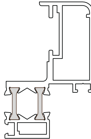
CEPHE İÇİ KANAT 5117 1,200 kg/m Jx: 19,90 cm 4 Jy: 3,68 cm 4 (Siyah Eloksal)
