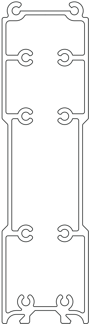
BAĞLANTI PROFİLİ 5127 0,467 kg/m
