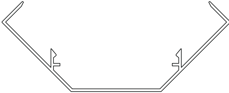
DIŞ KÖŞE KAPAK 5100 0,752 kg/m
