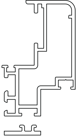
PANO PROFİLİ 5115 1,023 kg/m Jx: 14,14 cm 4 Jy: 3,33 cm 4 (Siyah Eloksal)
