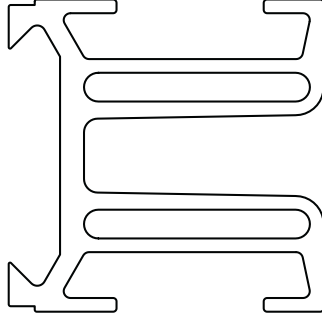
BAĞLANTI PROFİLİ 5126 1,672 kg/m
