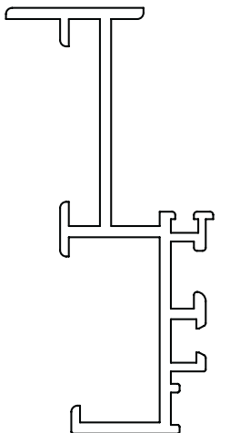
KOMPOZE PANO PROFİLİ 5119 0,770 kg/m Jx: 14,35 cm 4 Jy: 1,07 cm 4
