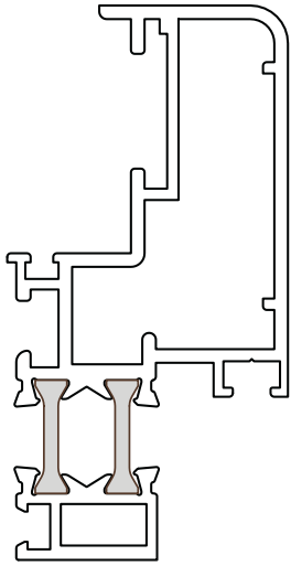
İZOLASYONLU PANO PROFİLİ 5116 1,289 kg/m Jx: 24,915 cm 4 Jy: 4,34 cm 4 (Siyah Eloksal)
