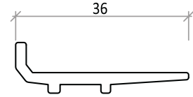
CAM TAKOZU PROFİLİ 5056 0,267 kg/m (Cam Kalınlığı 32mm'e Kadar)
