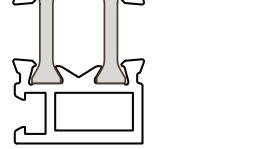
CAM YAPIŞTIRMA PROFİLİ 5120 0,279 kg/m (Siyah Eloksal)
