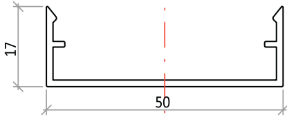
KAPAK PROFİLİ 5051 0,324 kg/m
