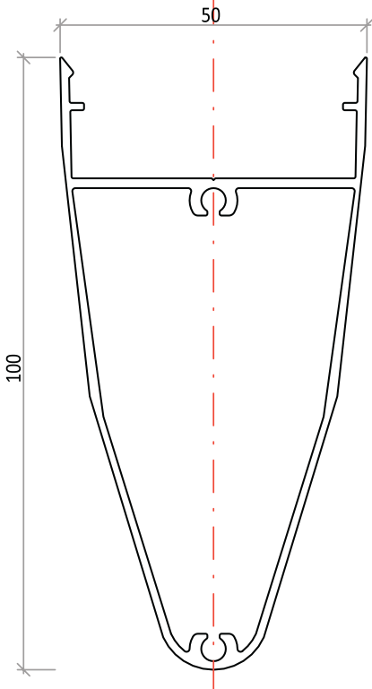
KAPAK PROFİLİ 5050 1,143 kg/m
